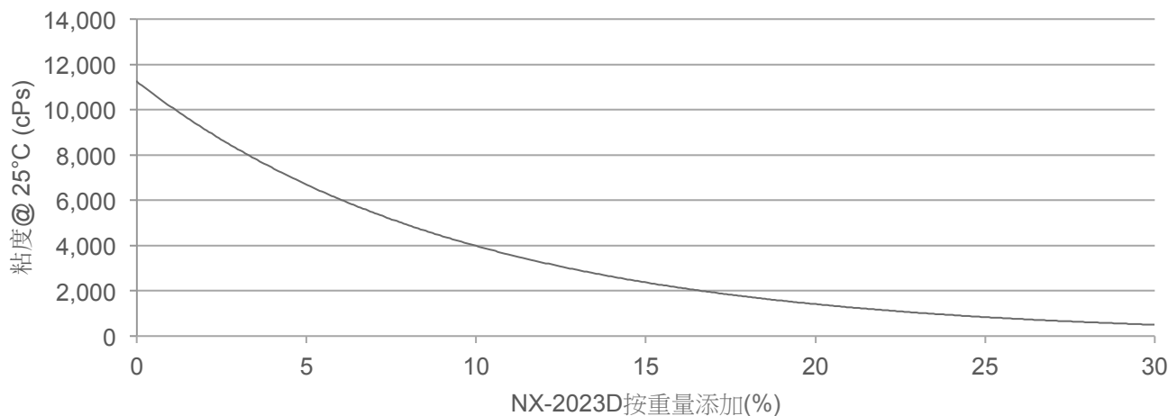
NX-2023D与液体环氧树脂混合的稀释曲线图（环氧当量=190）
